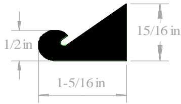
PFAUDLER #3200650 16" ID X 18 5/8" OD
