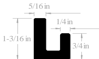
DAMROW #T-564-J-2 18-3/8" ID x 20-1/4" OD
